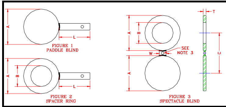
150# ANSI FLANGE RATING
